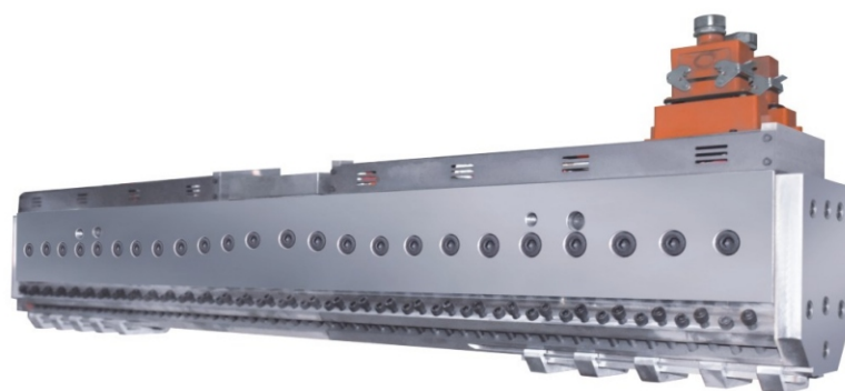
模具4 Mold 4
